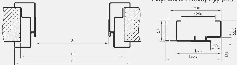
Profil ościeżnicy stalowej regulowanej z kątownikiem dymkającym T57
