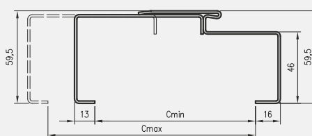
profil ościeżnicy
