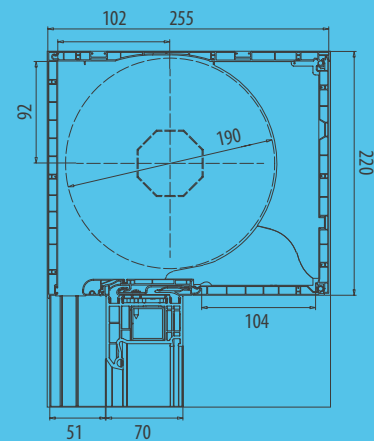
Skrzynka 220/255
