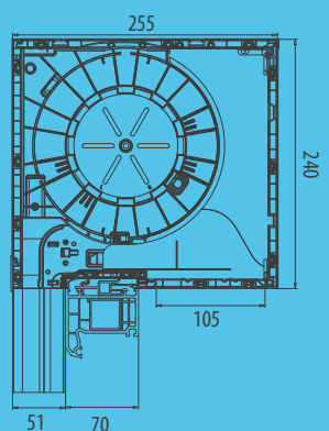
Skrzynka 240/255
