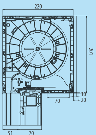
Skrzynka 201/220
