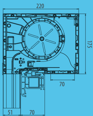
Skrzynka 175/220
