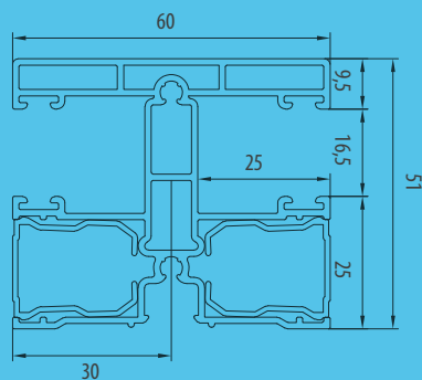
Odpowiednik aluminiowy
