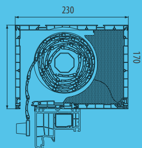
Skrzynka 170/230
