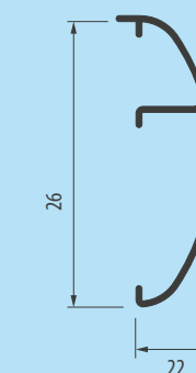
PPDO zaokrąglona nakładka na prowadnicę
