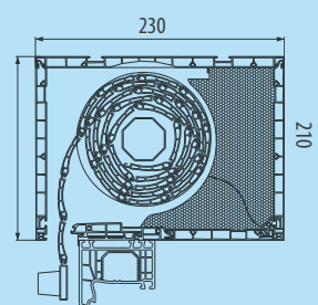
Skrzynka 210/230
