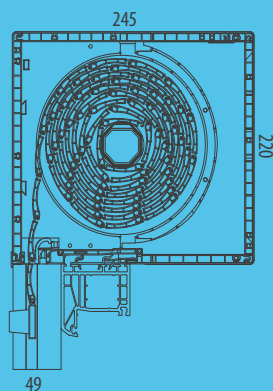
Skrzynka 220/245
