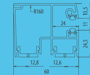
przewodnica R160 Aluminiowa przewodnica systemu EXTE EXAKT.
