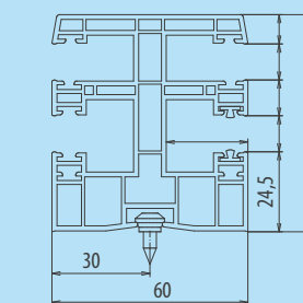
przewodnica R163 Przewodnica do rolety ze zintegrowaną moskitierą. Stosowane wkręty - RD1
