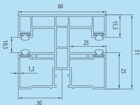
Prowadnica podziałowa
