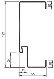
Ościeżnica stalowa S15/54
