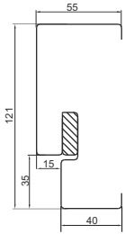
Ościeżnica stalowa T/54, T/54 AKU
