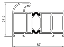
Profil ościeżnicy ALU/75
