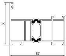
Profil naświetla
