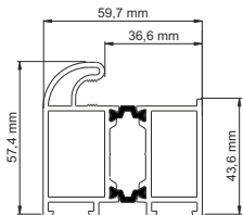
Profil ościeżnicy ALU/54
