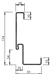
Ościeżnica stalowa 11/54, 11/54 ALU
