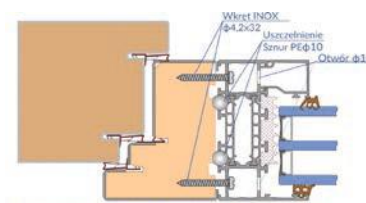
połączenie ościeżnicy z doświetlem aluminiowym
